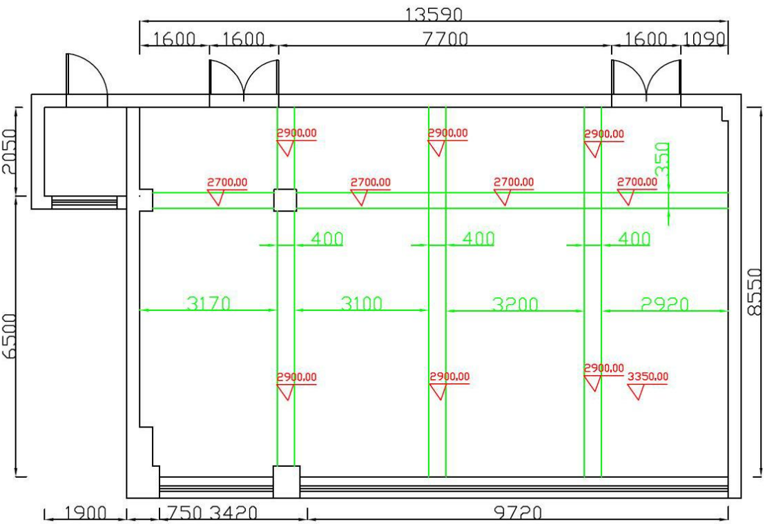
图 1-7 三楼会议室原始梁布置图
