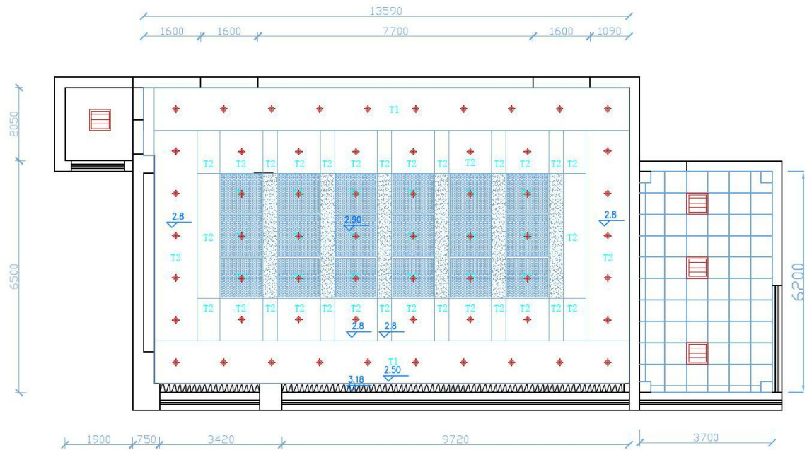
图 1-5 四层会议室顶部图
