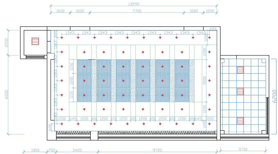
图 1-6 四层会议室顶面定位图
