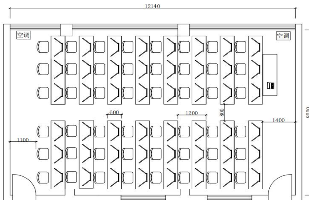
平面布置图
